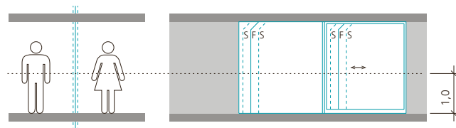
1-Meter-Regel: Personenschutz durch Sicherheitsglas (S); z. B. bei Festverglasungen, Hebeschiebe-, Schiebe- und Fenstertüren
